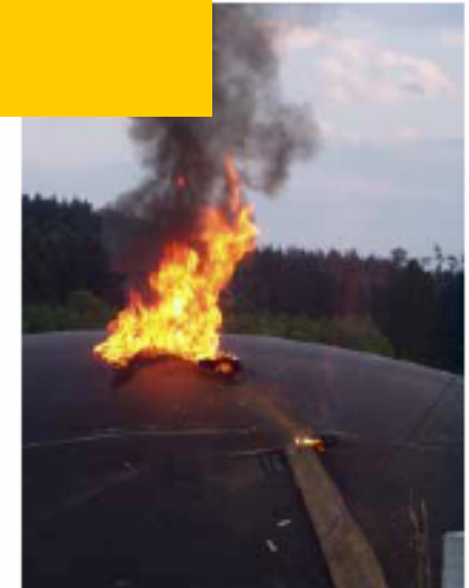
Bild 10 + 11: 6. Brandversuch ein brennender benzingertränkter Lappen wird auf den Foliengasspeicher geworfen
